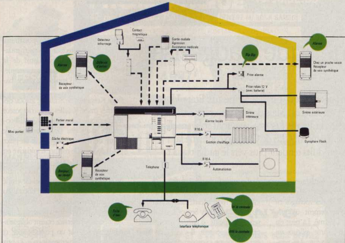
Le plan complet des fonctions du Securiscan, qui résume bien ce qu'est aujourd'hui la domotique. Les traits pointillés symbolisent les liaisons par ondes, les traits pleins les liaisons électriques. Le contrôle par téléphone (et non pas le seul passage d'ordres) est un atout du système Thomson.
